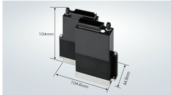
RICOH TH6310F
